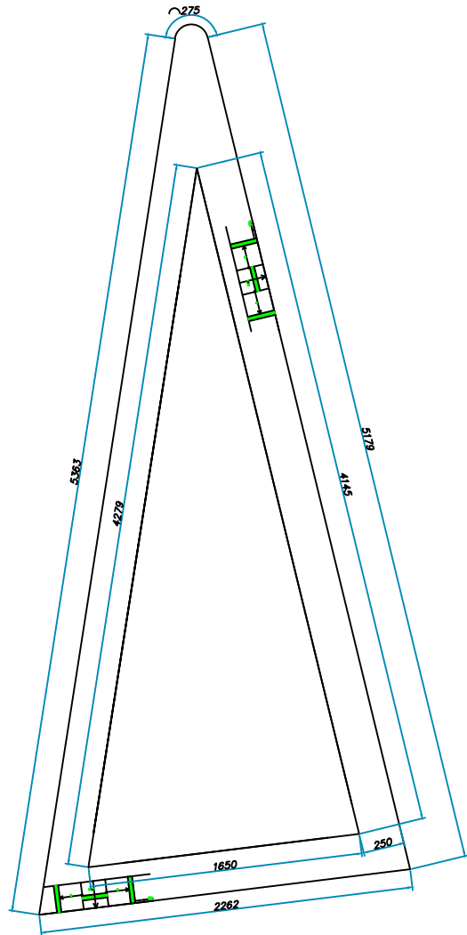
PLANTA LOCAÇÃO ESC. 1/200
