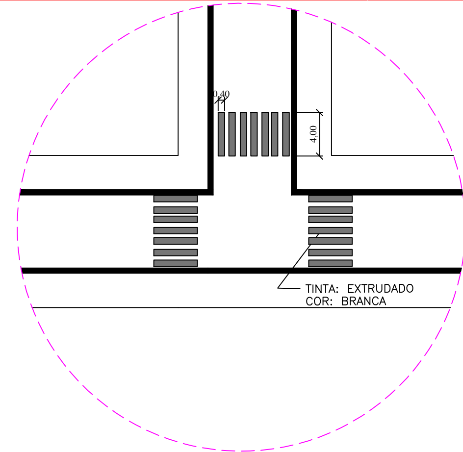
DET.1 – FAIXA DE PEDESTRE SEM ESCALA
