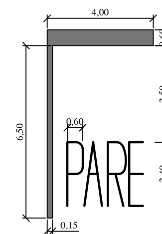
DET.2 – DESENHO TIPO SH – "PARE" SEM ESCALA
